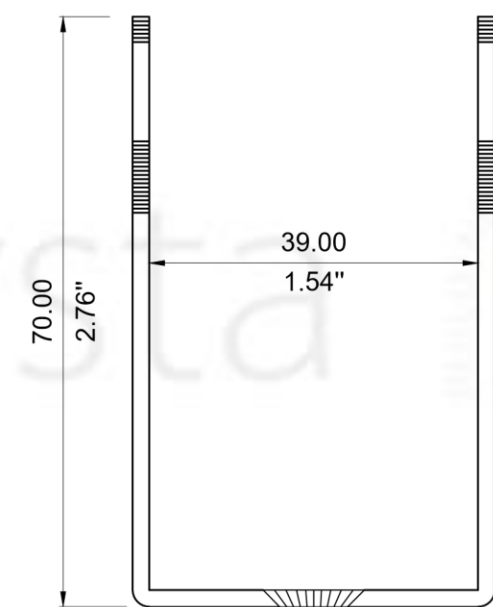
3 FRONT ELEVATION U-3 N.T.S
