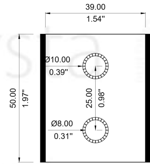
2 PLAN U-2 N.T.S
